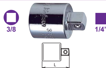
RACCORDO DI RIDUZIONE QUADRO MASCHIO 1/4" E FEMMINA 3/8"
