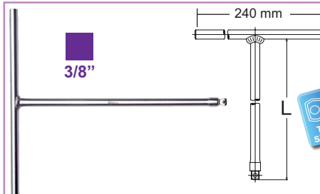
CHIAVI A "T" MASCHIO QUADRO 3/8" TESTA SFERICA CON IMPUGNATURA LARGHEZZA 240 MM
