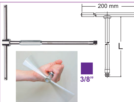
CHIAVI A "T" MASCHIO QUADRO 3/8" CON ASTA SCORREVOLE E CANOTTO DI ROTAZIONE LARGHEZZA 200 MM
