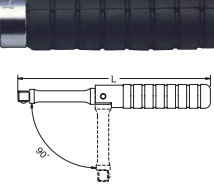
QUADRO MASCHIO PIEGHEVOLE 90° CON IMPUGNATURA
